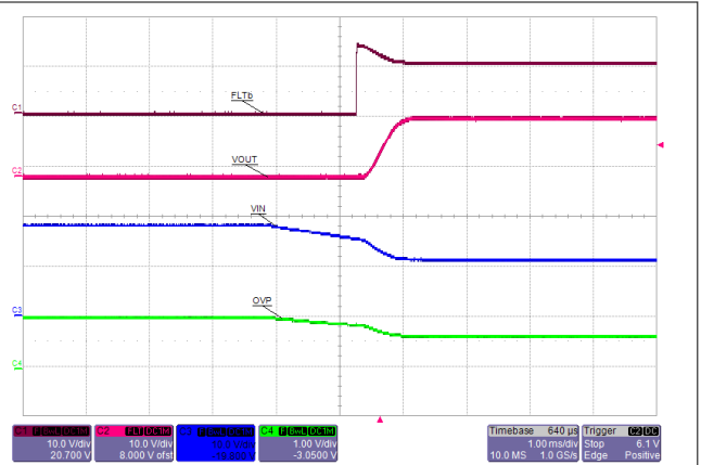
图 10-10. Overvoltage Recovery
