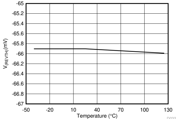
图 7-29. V (REVTH) vs Temperature
