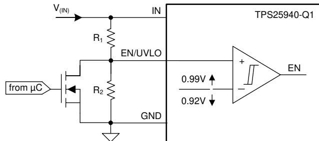
图 9-8. Shutdown Control
