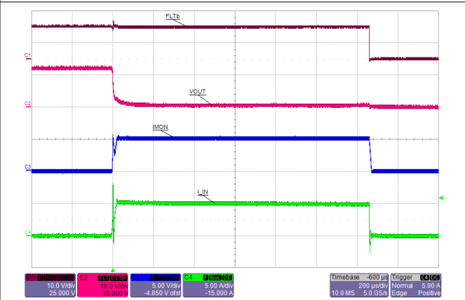
图 10-18. Hot Short: Latched - TPS25940L-Q1
