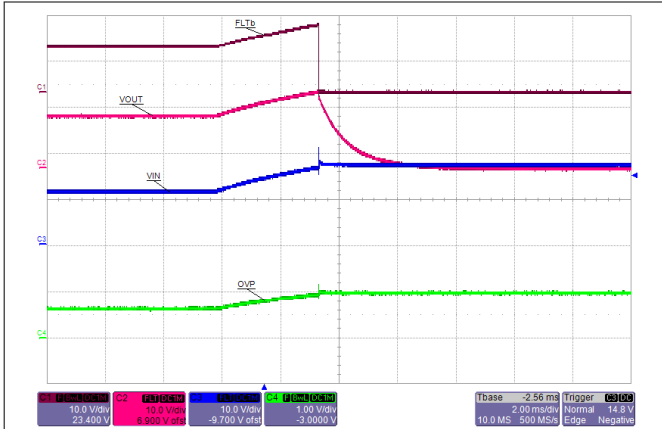
图 10-9. Overvoltage Shutdown
