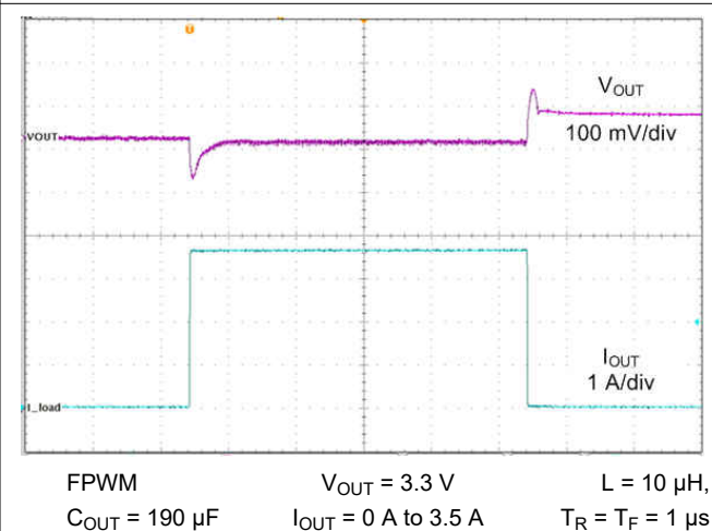
图 9-28. Load Transient
