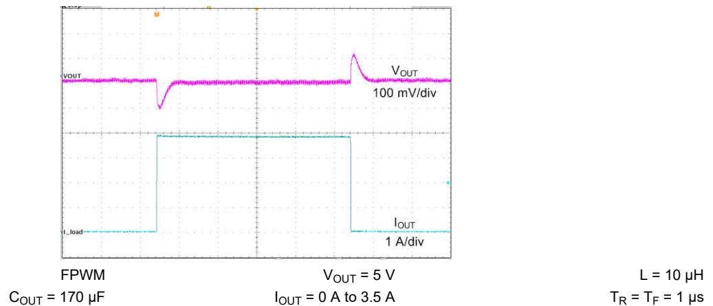
图 9-15. Load Transient
