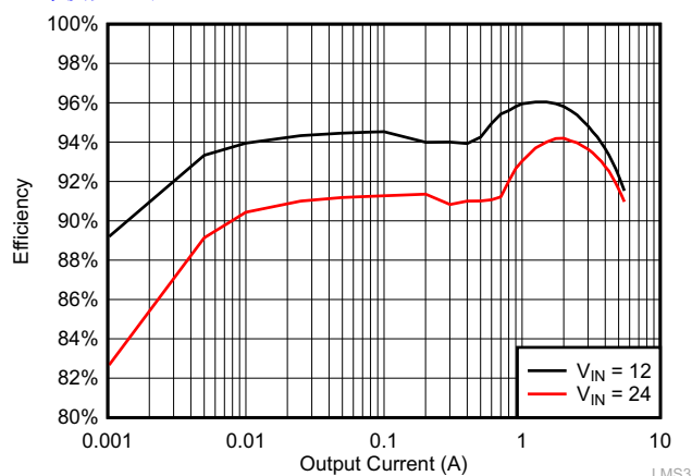
LMS3655-Q1 效率： V_{OUT} = 5V
