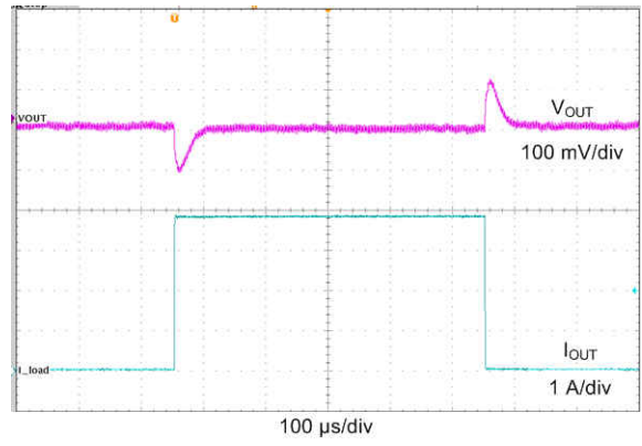
图 9-33. Load Transient
