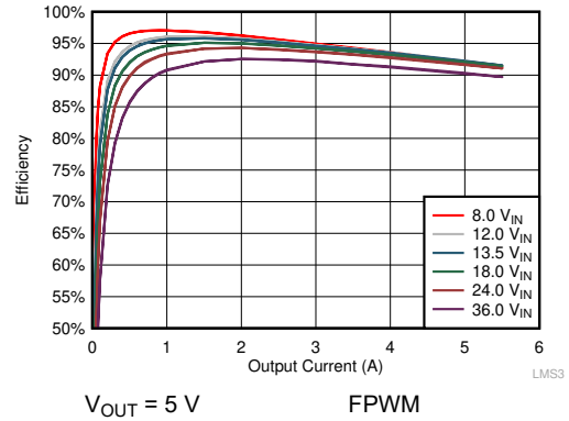
图 9-6. Efficiency
