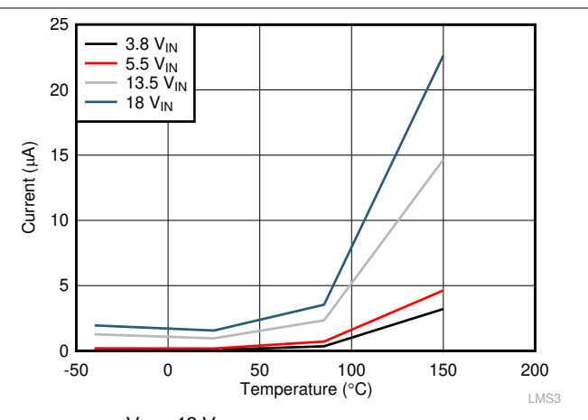
图 7-6. Shutdown Current
