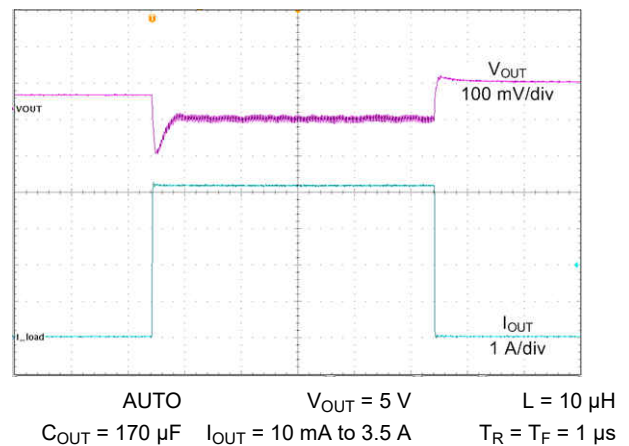
图 9-14. Load Transients
