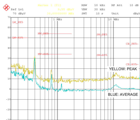
LMS3655-Q1 传导 EMI： V_{OUT} = 5V ， I_{OUT} = 5A
