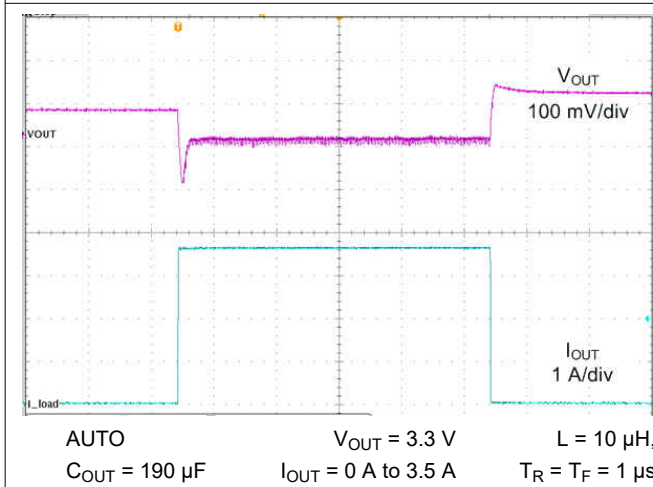
图 9-27. Load Transient
