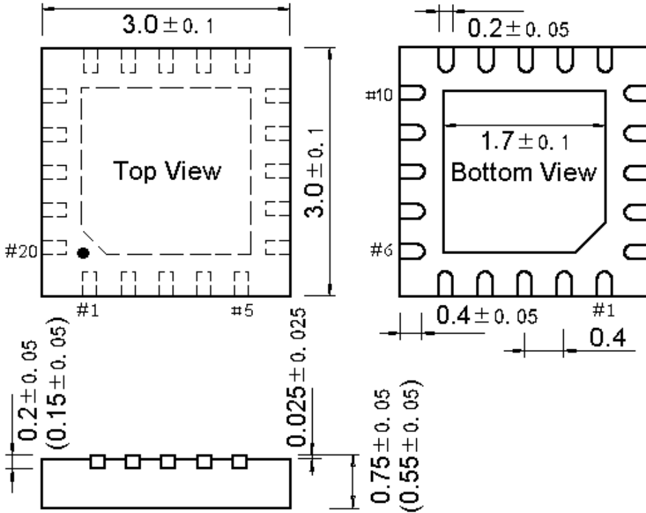
图 4-2 QFN20 封装
