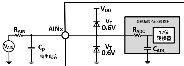
图 3-10 ADC 典型连接图
