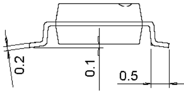
图 4-4 SOP8 封装
