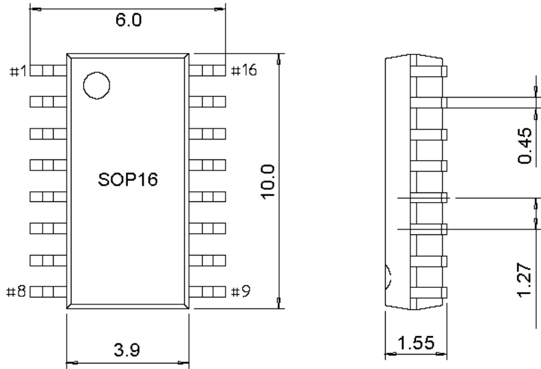
图 4-3 SOP16 封装
