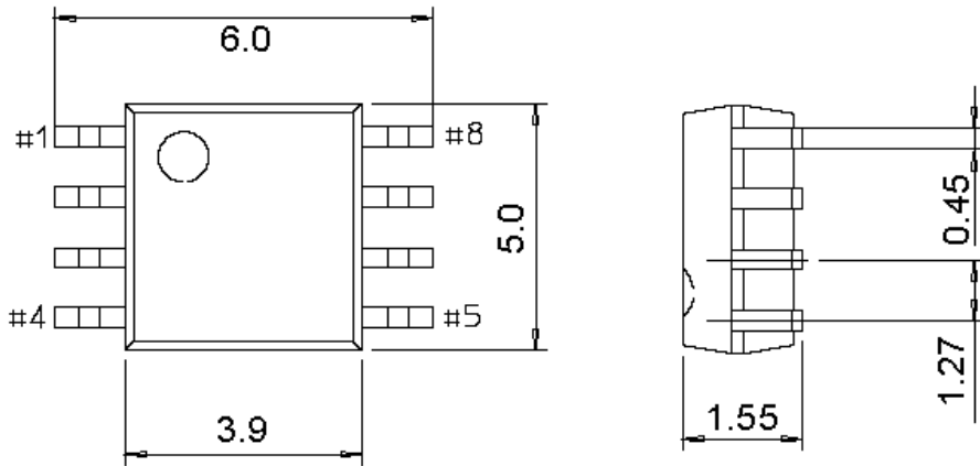
图 4-4 SOP8 封装
