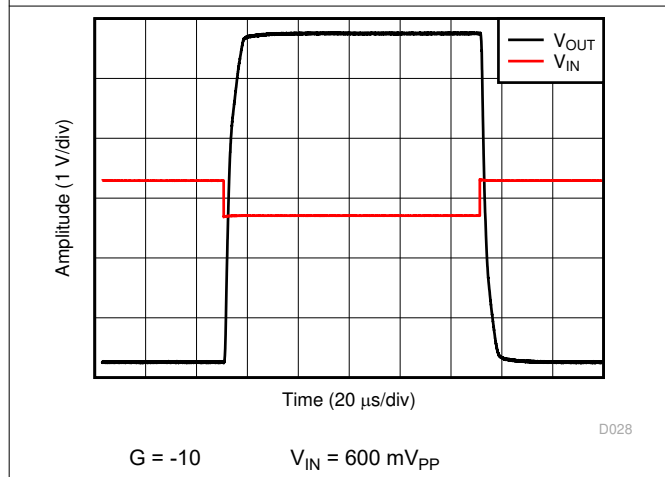
图 6-22. 过载恢复
