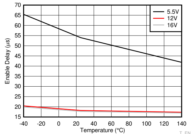
图 6-12. Enable Delay
