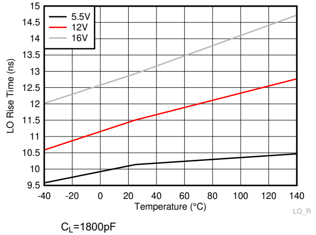
图 6-22. LO Rise Time
