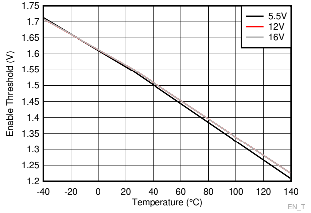
图 6-10. Enable Threshold
