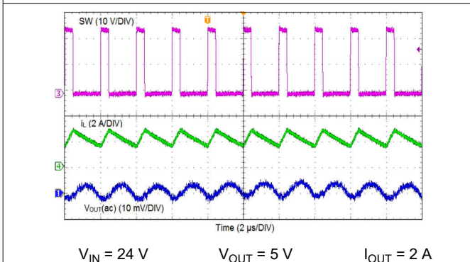
图 8-6. CCM Mode
