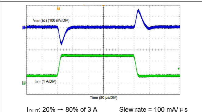
图 8-7. Load Transient
