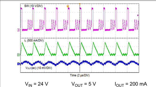
图 8-5. DCM Mode
