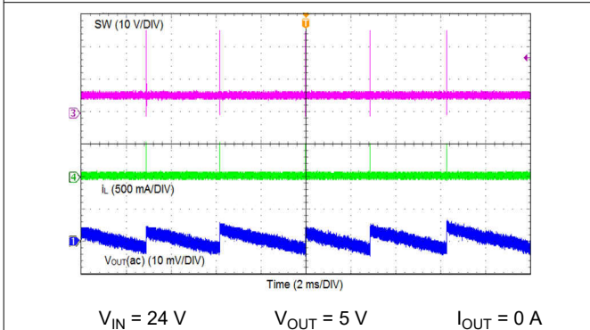
图 8-4. Sleep Mode
