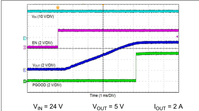
图 8-2. Start-up By EN
