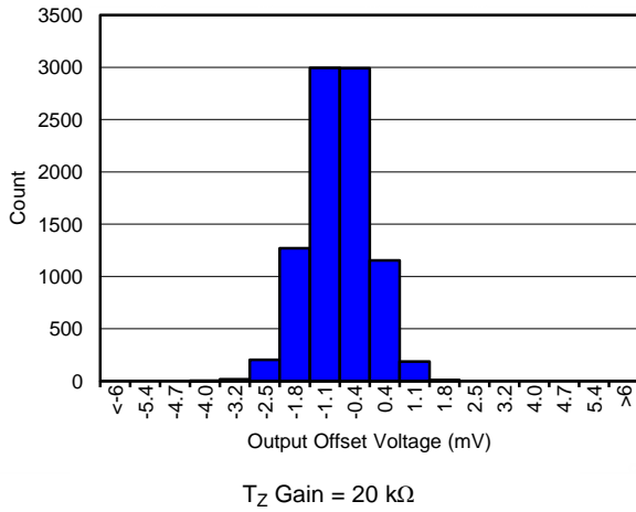
图 33. Differential V_{OsO} Histogram
