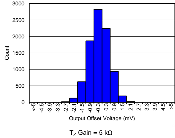
图 32. Differential V_{OsO} Histogram
