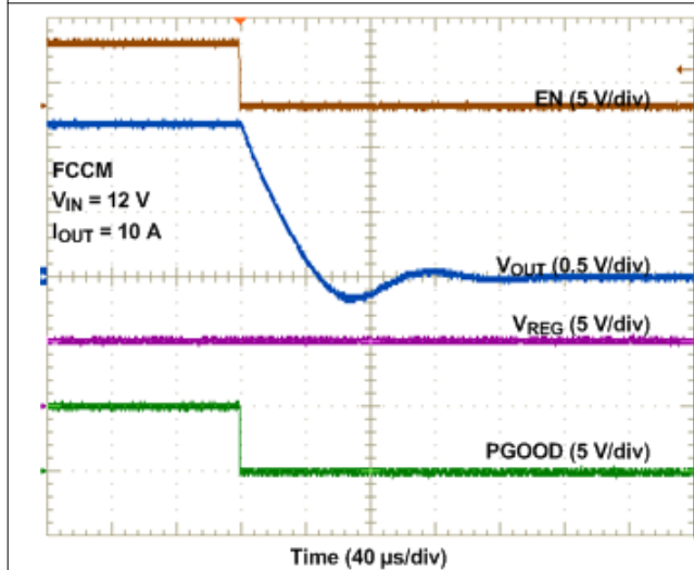
图 9-15. Shutdown
