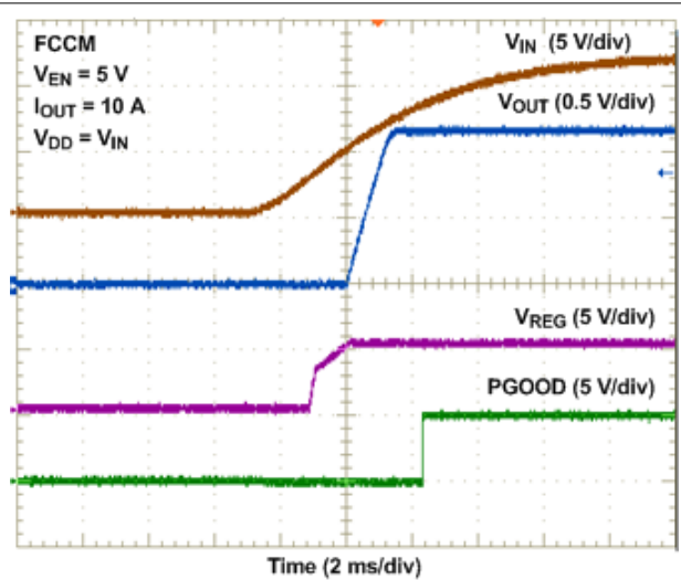
图 9-16. UVLO Start-Up
