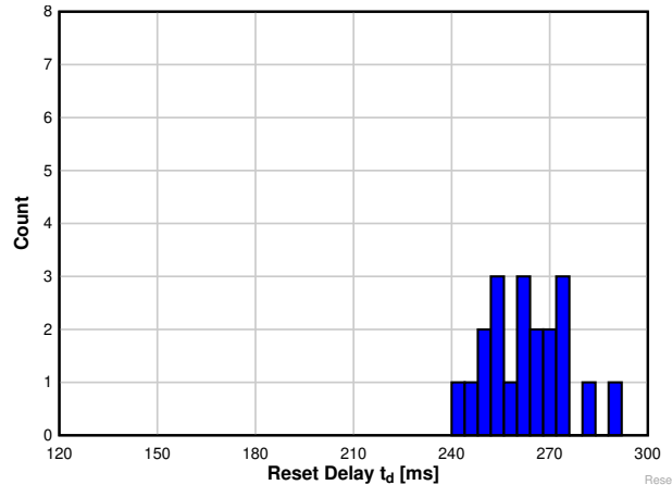
图 7-9. TPS3823A-33 器件在 -40^{\circ}\text{C} 时的复位延时直方图 (单位数 = 20)
