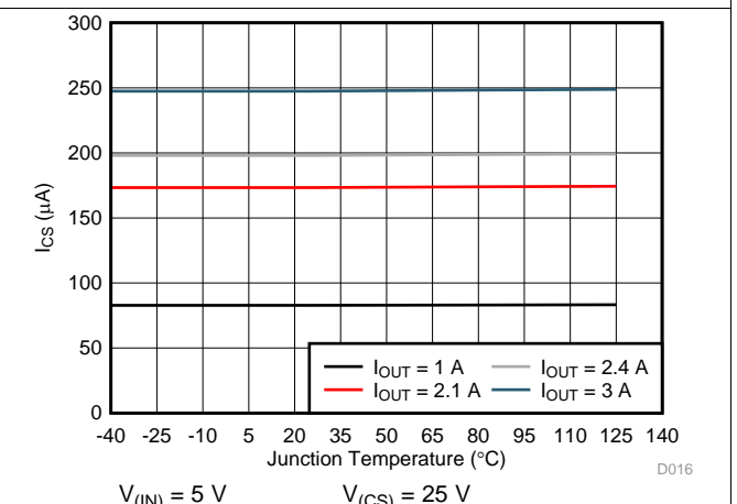
图 12. I_{(CS)} vs Temperature
