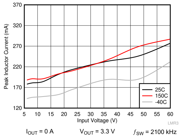
图 7-6. I_{PEAK-MIN}
