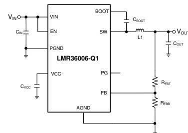
简化版原理图
