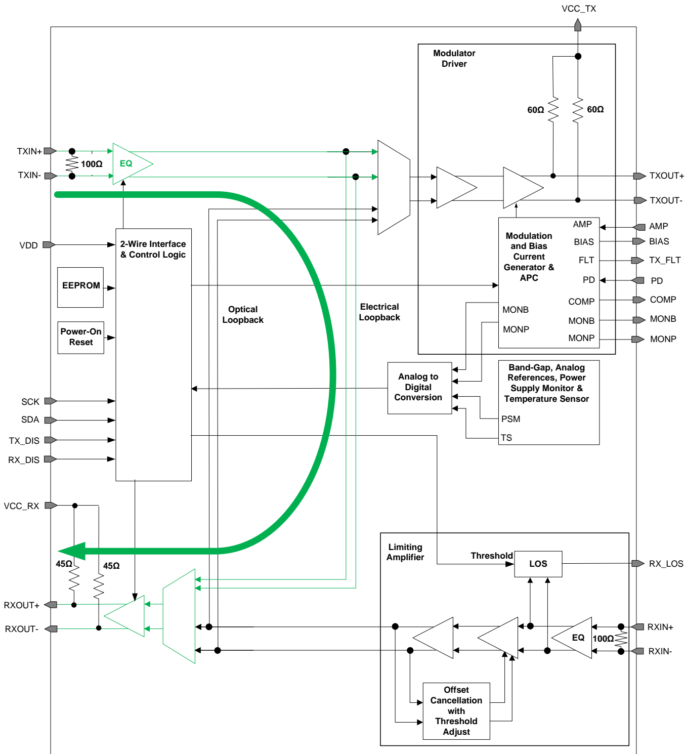
图 35. Electrical Loopback
