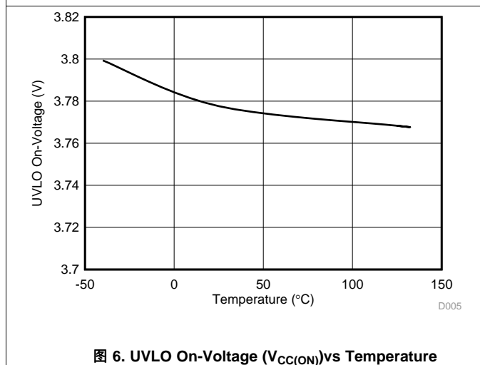
图 6. UVLO On-Voltage ( V_{\text{CC(ON)}} ) vs Temperature
