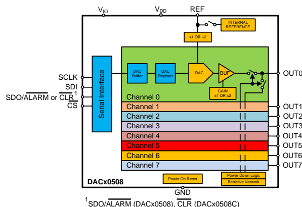
简化方框图
