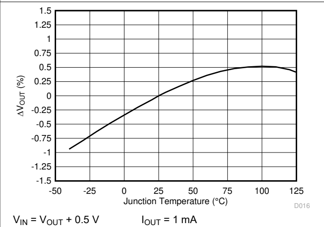
图 6-16. \Delta V_{OUT} vs Temperature
