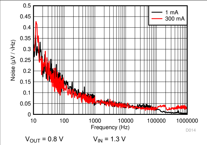
图 6-14. Noise Density
