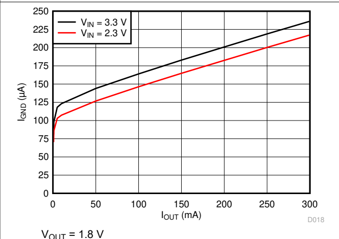
图 6-18. I_{GND} vs I_{OUT}
