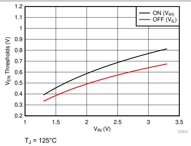
图 6-4. V_{EN} Thresholds vs V_{IN}
