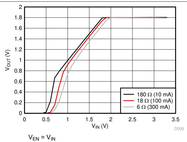
图 6-6. V_{OUT} vs V_{IN}
