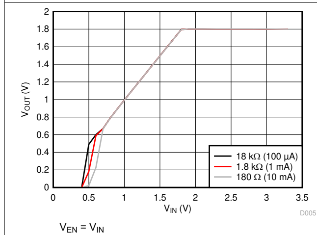
图 6-5. V_{OUT} vs V_{IN}
