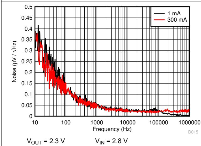
图 6-15. Noise Density
