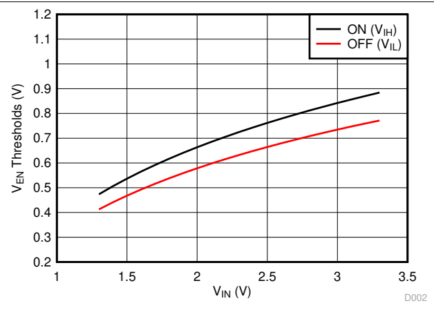
图 6-2. V_{EN} Thresholds vs V_{IN}
