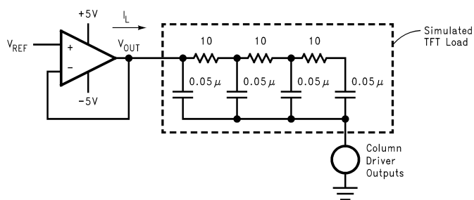
图 67. V_{COM} 驱动器应用原理图
