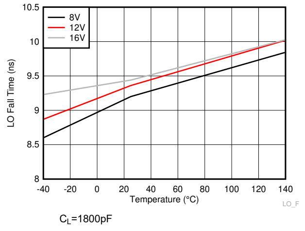
图 6-17. LO Fall Time
