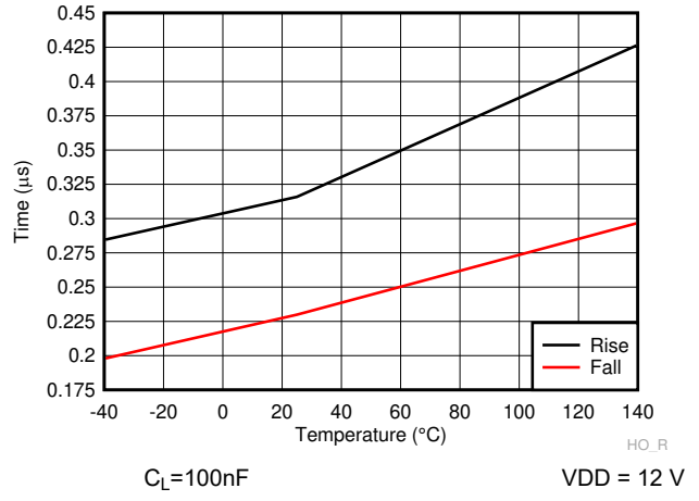
图 6-21. HO Rise & Fall Time
