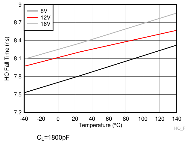
图 6-19. HO Fall Time
