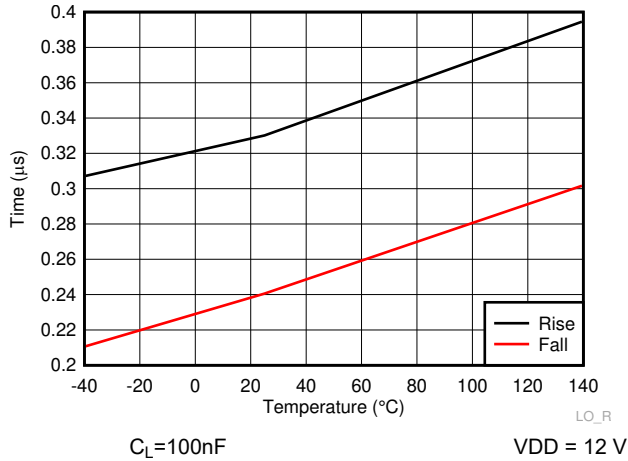
图 6-20. LO Rise & Fall Time
