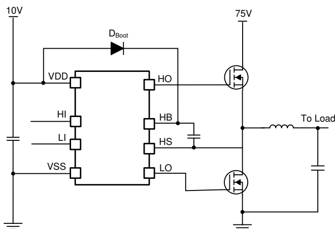
简化版应用图
