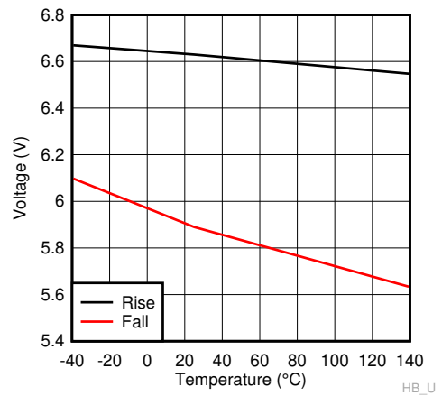
图 6-11. HB UVLO Threshold
