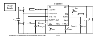
简化版电路原理图
