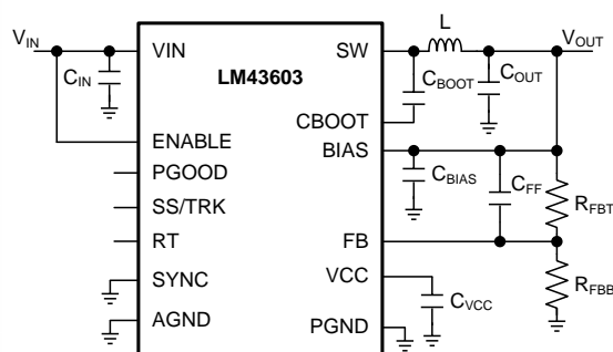
简化原理图
