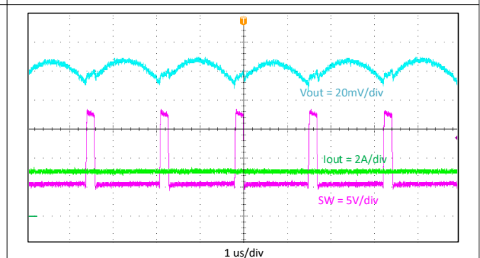
图 9-7. 输出电压纹波, I_{out} = 3A
