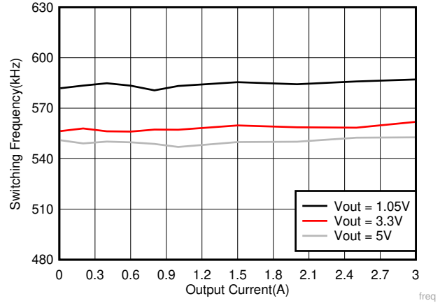
图 7-8. 开关频率与输出电流间的关系
