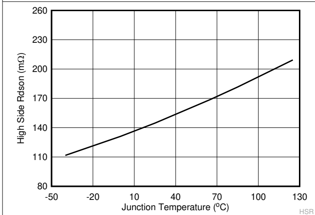
图 7-5. 高侧 R_{ds-On} 与结温间的关系
