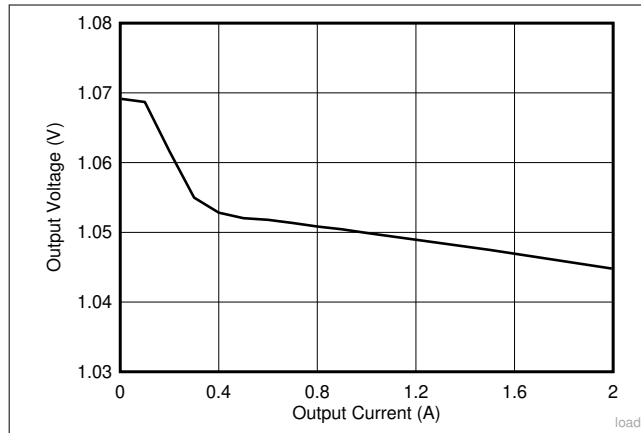
图 9-2. 不同负载的负载调节
