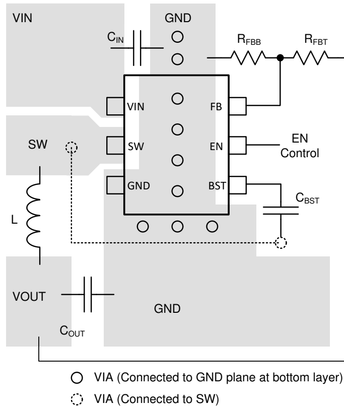
图 11-1. TPS562202 布局
