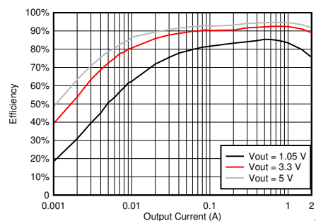
TPS562202 效率
