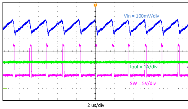
图 9-4. 输入电压纹波, I_{out} = 2A
