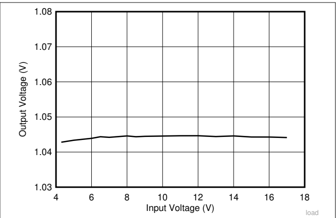
图 9-3. 不同输入电压的负载调节
