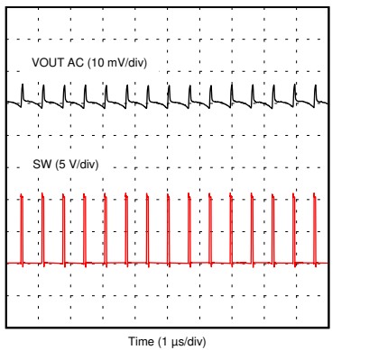
图 8-28. Output Ripple – No Load
