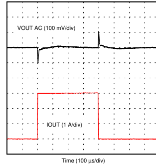
图 8-32. Load Transient
