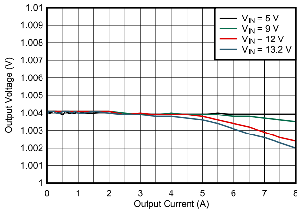
图 8-26. Load Regulation
