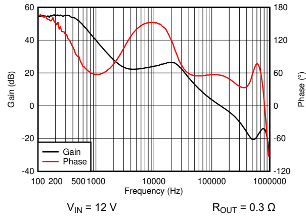
图 8-7. Bode Plot
