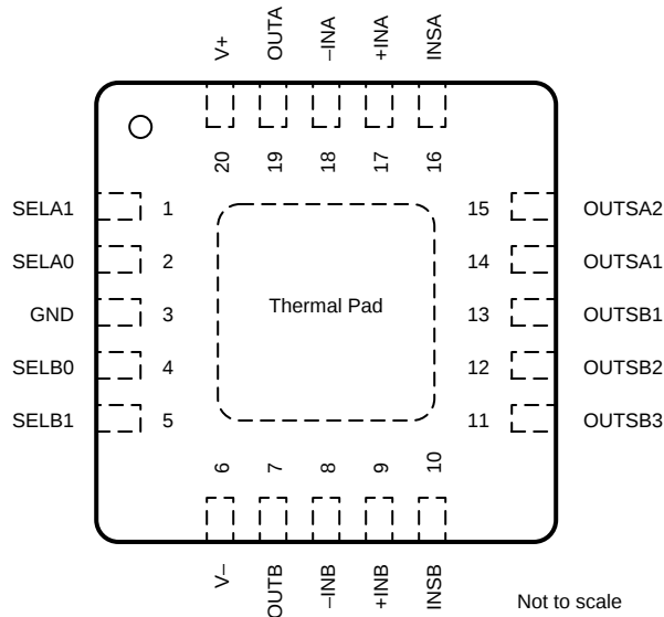
图 5-1. OPA3S328 RGR (20-Pin VQFN) Package, Top View
