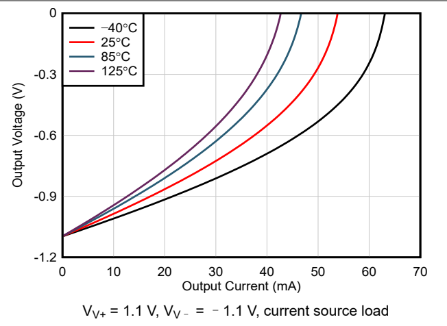
图 6-21. Output Voltage Swing vs Output Current
