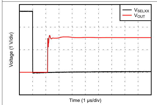
图 6-48. Switch Turn-on
