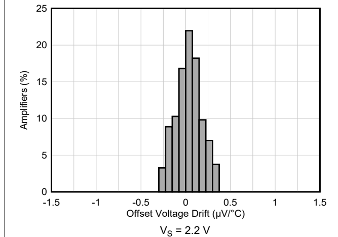
图 6-4. Offset Voltage Drift Distribution
