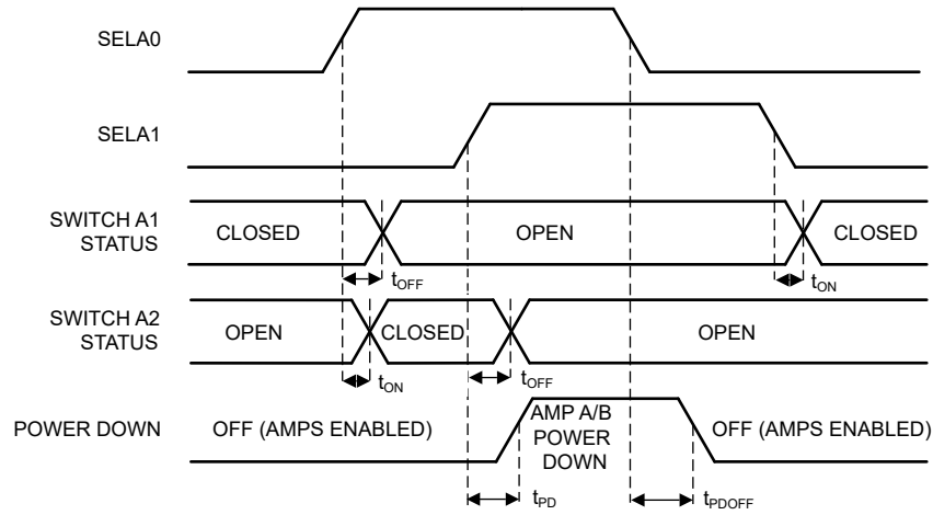
图 6-1. Select Pin Timing Diagram
