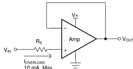
图 8-1. Input Current Protection
