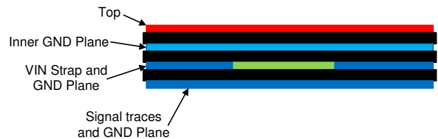
图 11-2. Example Layout for VQFN Package
