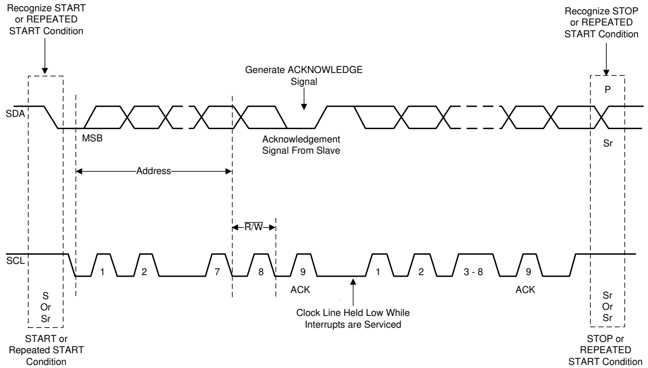
图 8-22. Bus Protocol
