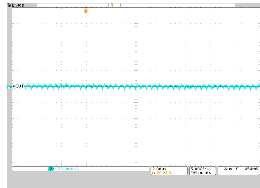
图 10-45. Output Voltage Ripple
