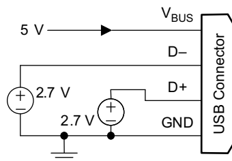
图 10-17. Divider 3 Mode
