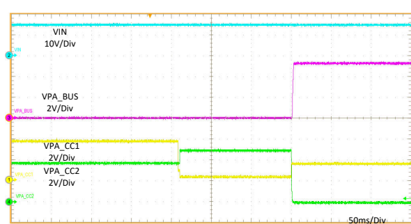
图 11-18. Startup Relate to EN
