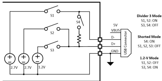
图 10-19. DCP Auto Mode
