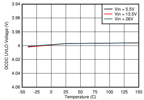
图 8-6. DCDC UVLO Threshold
