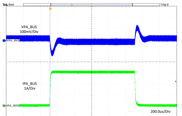
图 11-5. Load Regulation
