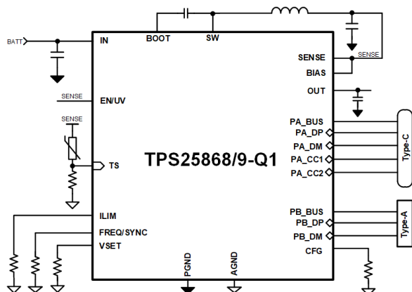
简化版原理图：TPS2586x-Q1
