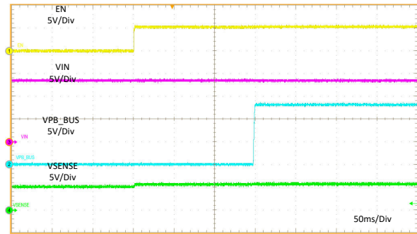
图 11-18. Startup Relate to EN
