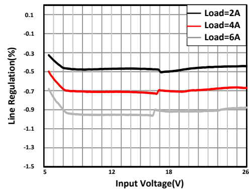
图 11-6. Line Regulation
