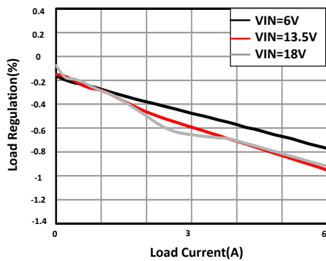
图 11-5. Load Regulation
