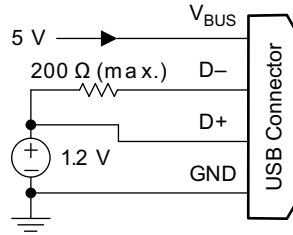
图 10-18. 1.2-V Mode
