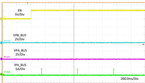
图 11-21. Rd Assert
