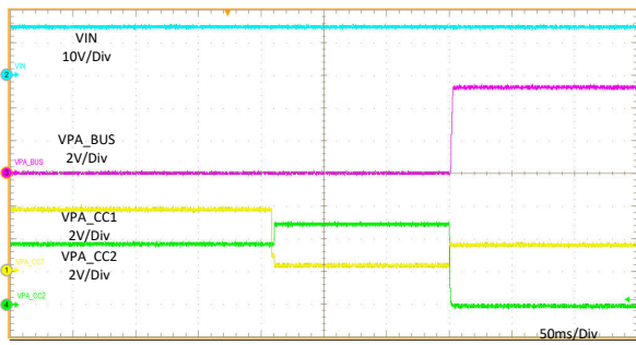
图 11-21. Rd Assert
