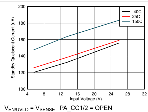
图 8-2. Standby Quiescent Current
