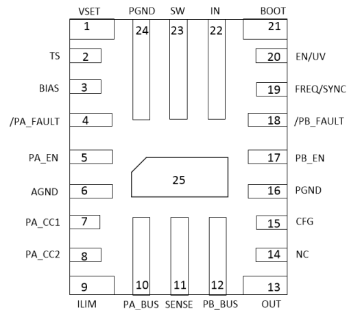
图 7-2. TPS25862 RPQ Package 25-Pin (QFN) Top View
