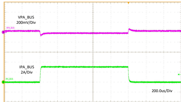
图 11-6. Load Regulation
