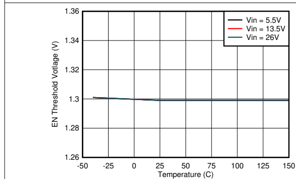
图 8-3. Precision Device Enable Threshold
