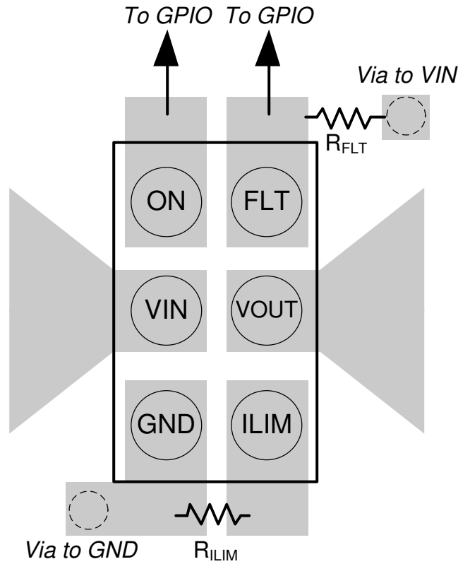
图 12-1. TPS22950x Layout Example
