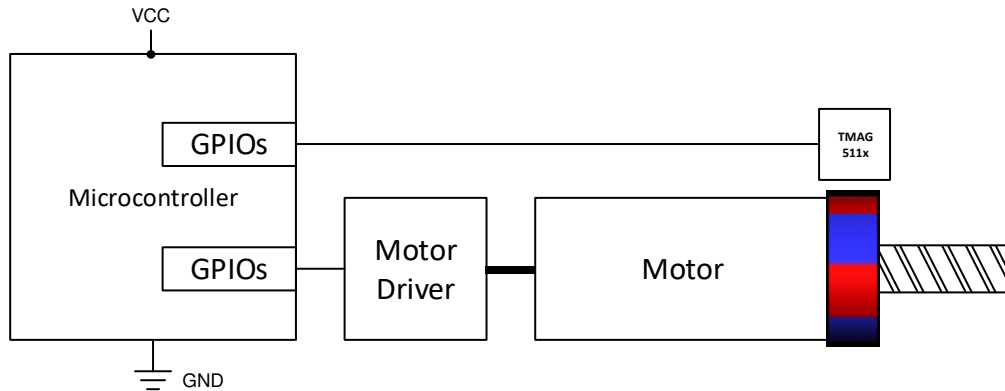
图 9-1. 增量编码
