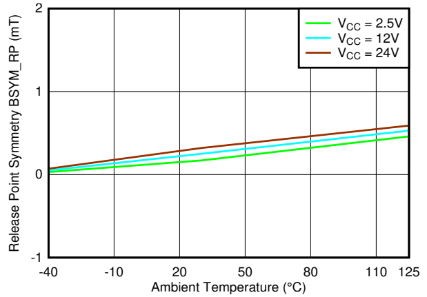
图 7-66. B_{SYM\_RP(ZX)} 与温度
