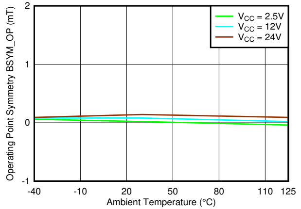
图 7-64. B_{SYM\_OP(ZX)} 与温度
