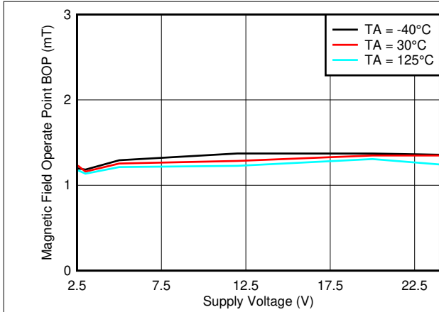
图 7-1. B OP_Z 阈值与 V CC
