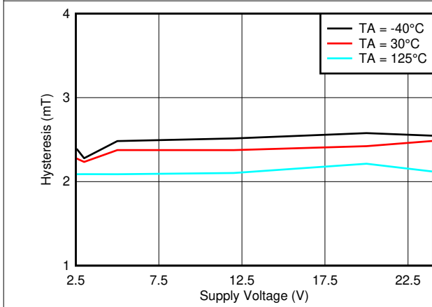
图 7-5. Hysteresis Z 与 V CC
