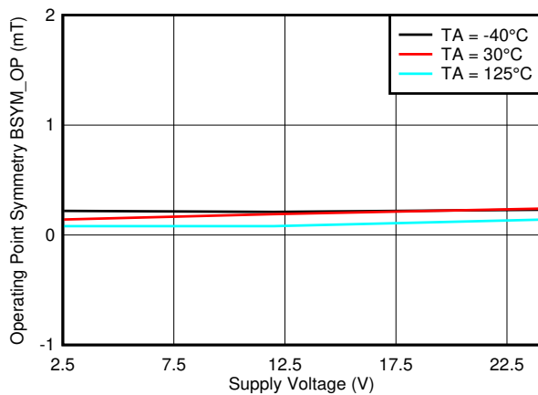
图 7-67. B_{SYM\_OP(ZY)} 与 V_{CC}
