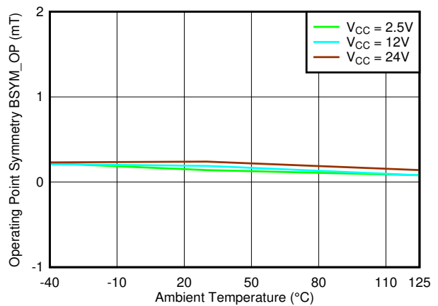
图 7-68. B_{SYM\_OP(ZY)} 与温度
