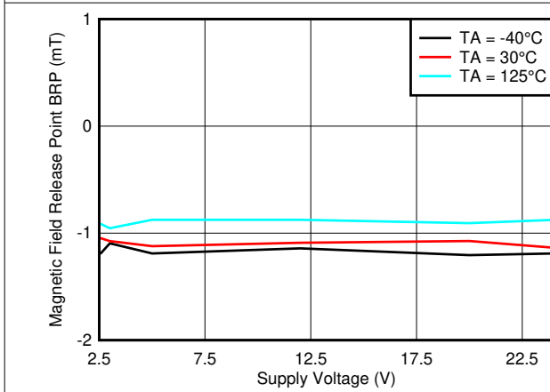
图 7-3. B RP_Z 阈值与 V CC
