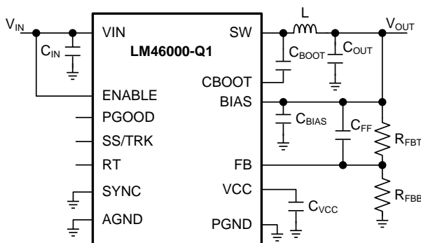
简化原理图
