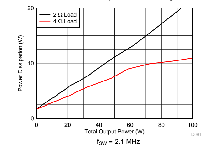
图 30. Power Dissipation vs Total Output Power
