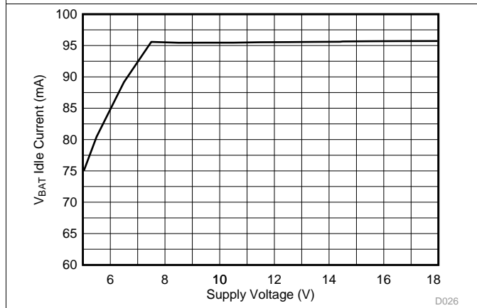
图 17. VBAT Idle Current vs Voltage
