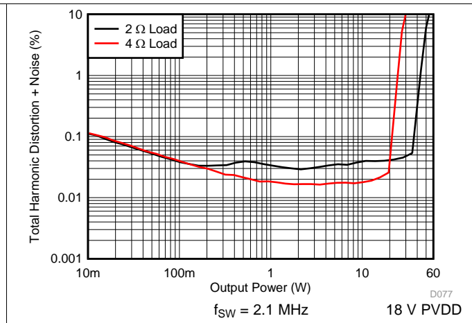
图 26. PBTL THD+N vs Power
