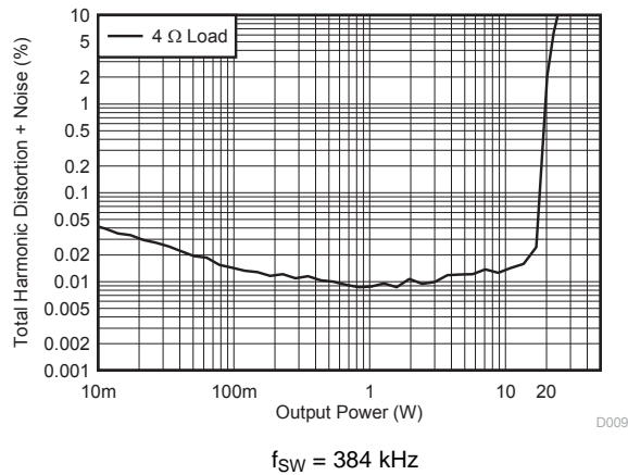
图 7. THD+N vs Power
