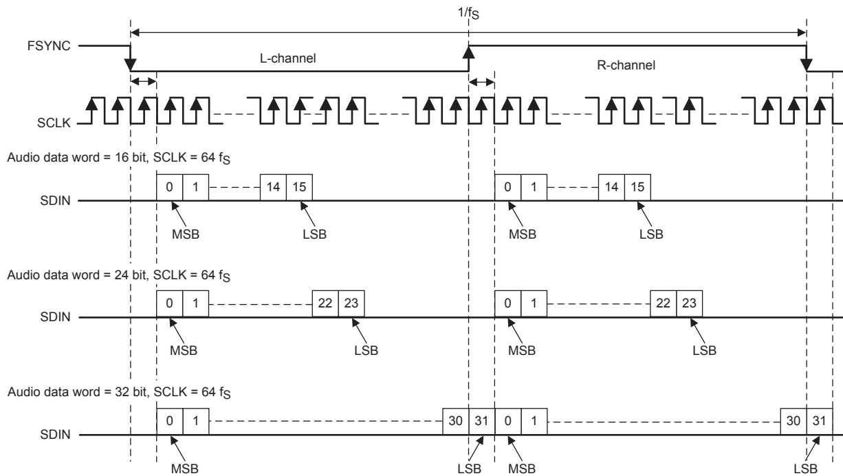
图 34. I²S Audio Data Format
