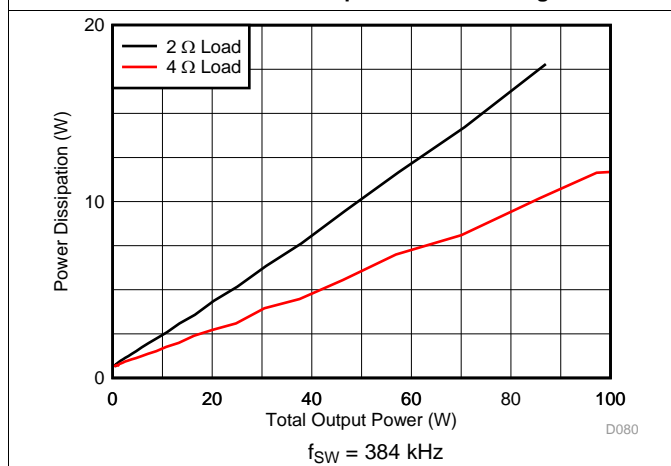
图 29. Power Dissipation vs Total Output Power
