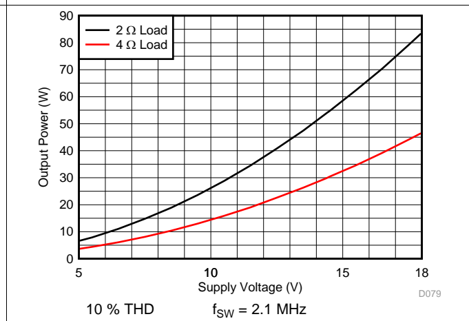
图 28. PBTL Output Power vs Voltage
