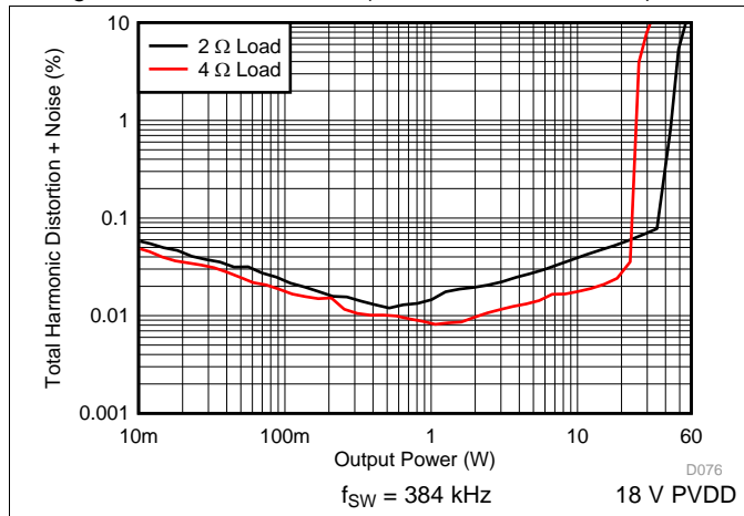
图 25. PBTL THD+N vs Power
