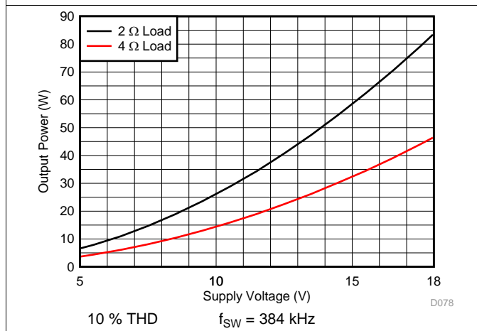
图 27. PBTL Output Power vs Voltage
