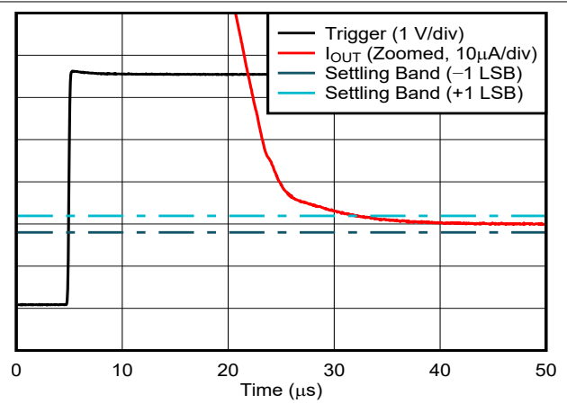
图 6-44. 电流输出建立时间 (下降沿)
