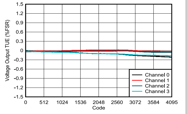
图 6-13. 电压输出 TUE 与数字输入代码间的关系
