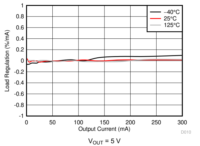
图 6-10. Load Regulation
