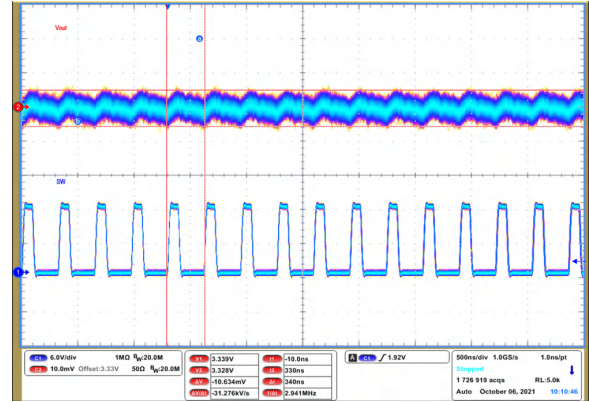
图 9-75. Output Voltage Ripple
