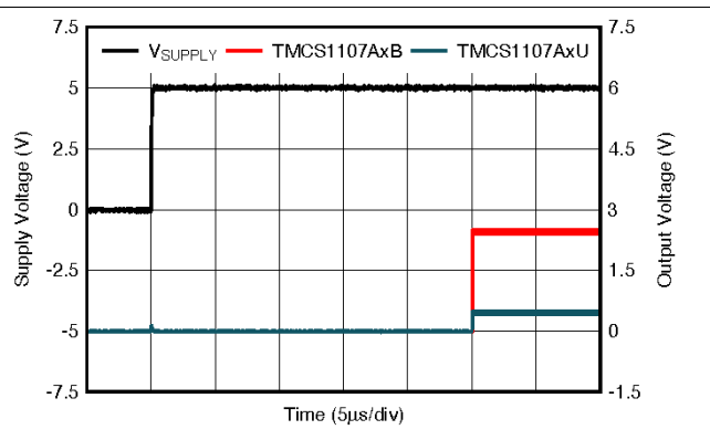
图 7-12. 启动瞬态响应
