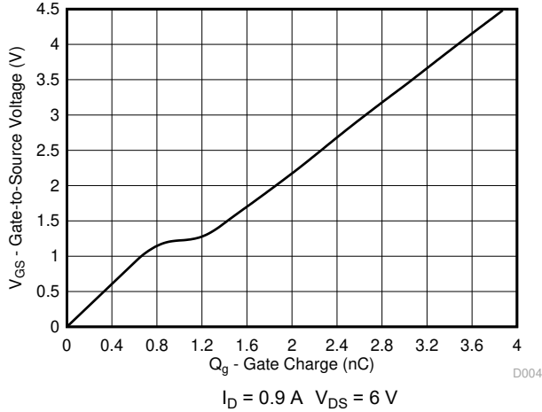
图 5-4. Gate Charge
