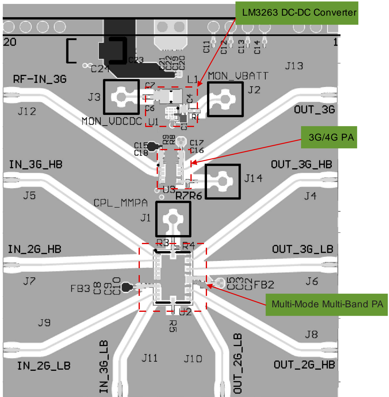
Figure 29. 具有 PA 的 RF 评估板顶视图
