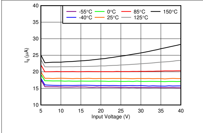
图 6-27. Quiescent Current ( I_Q ) vs V_{IN}
