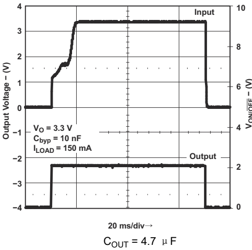
图 8-23. Turn-On Time
