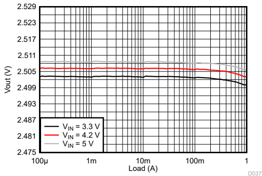
图 9-43. Load Regulation
