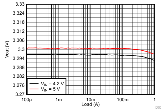
图 9-44. Load Regulation
