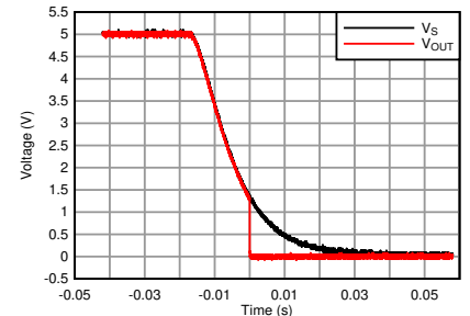
图 37. TLV4041/4051 Output for V_S Falling
