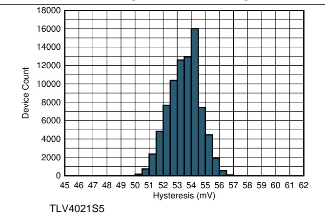
图 20. Hysteresis Histogram
