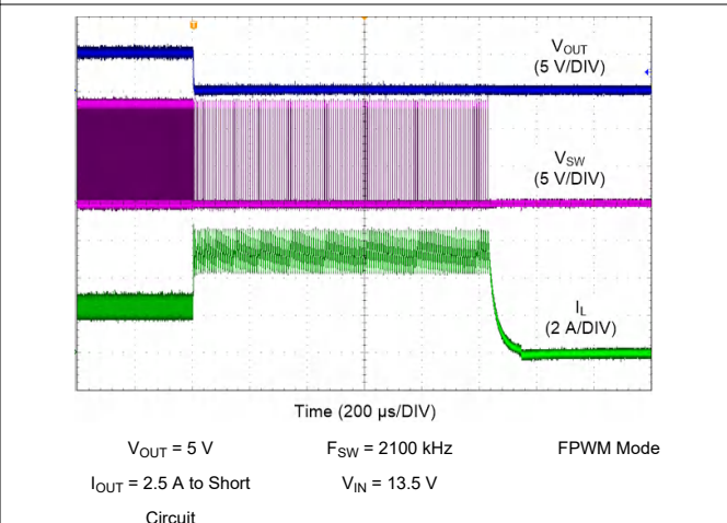
图 9-20. LM62435-Q1 Short Circuit Protection
