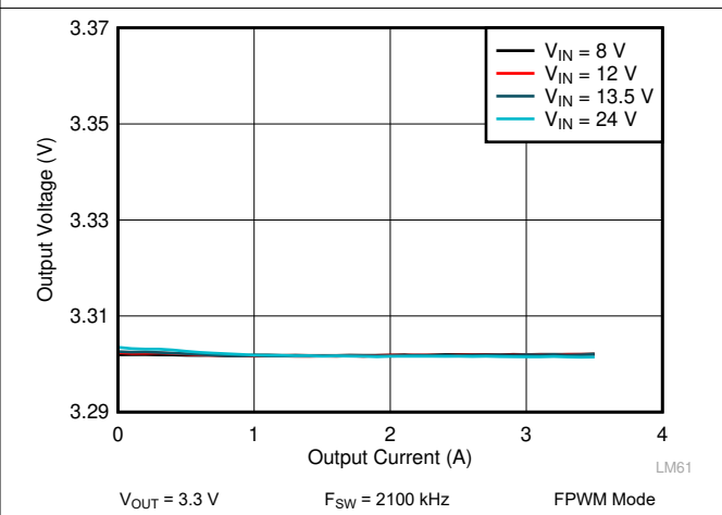
图 9-10. LM62435-Q1 Load and Line Regulation
