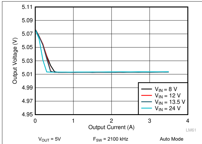
图 9-11. LM62435-Q1 Load and Line Regulation
