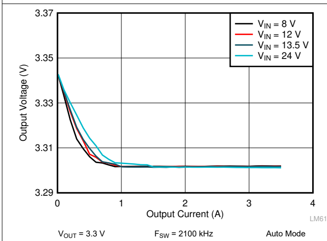
图 9-9. LM62435-Q1 Load and Line Regulation
