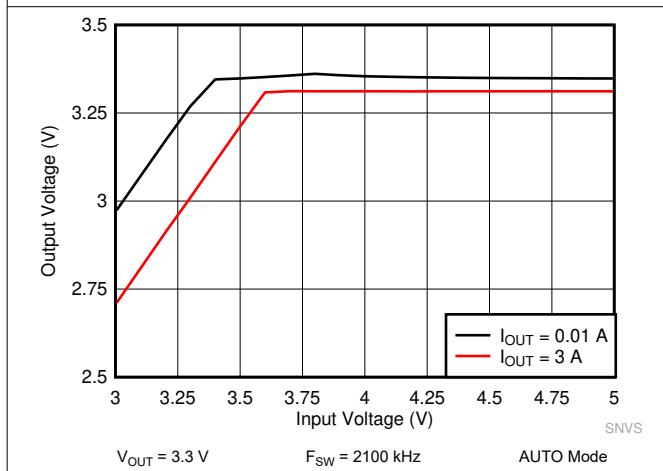
图 9-13. LM62435-Q1 Dropout Curve
