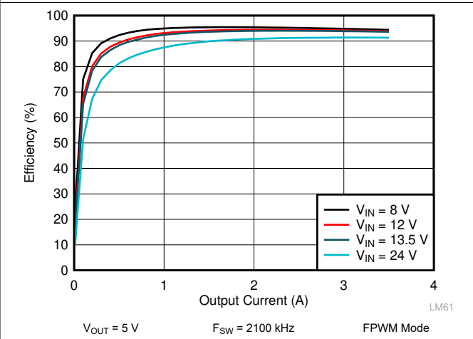
图 9-8. LM62435-Q1 Efficiency
