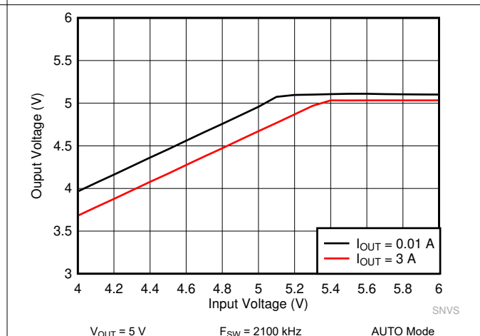
图 9-14. LM62435-Q1 Dropout Curve
