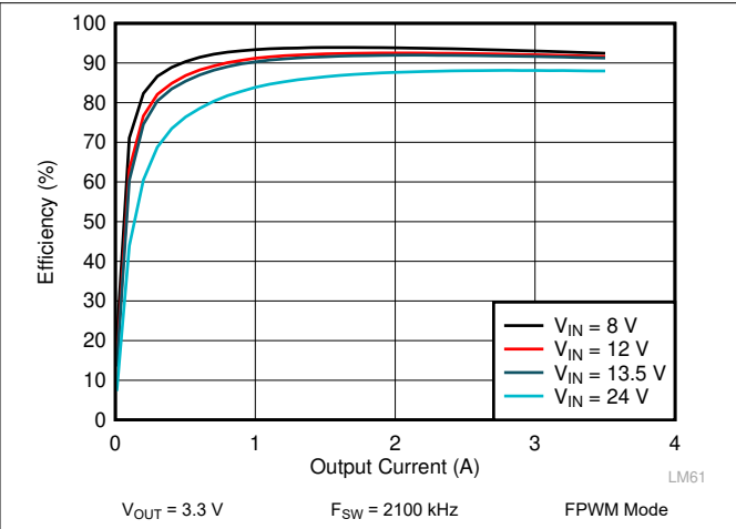
图 9-6. LM62435-Q1 Efficiency
