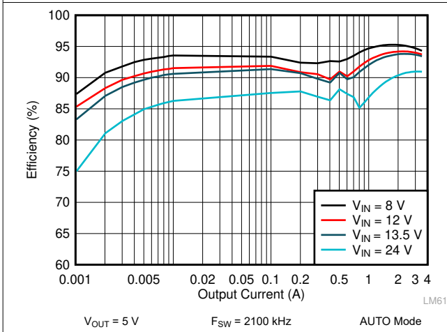
图 9-7. LM62435-Q1 Efficiency
