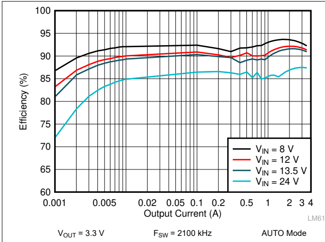
图 9-5. LM62435-Q1 Efficiency
