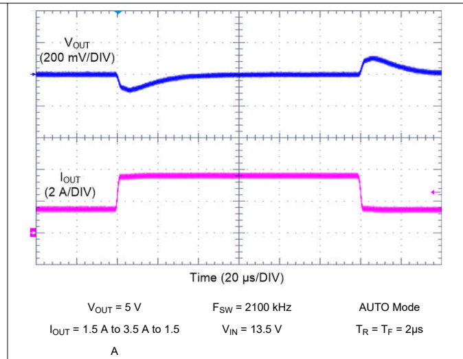
图 9-24. LM62435-Q1 Load Transient
