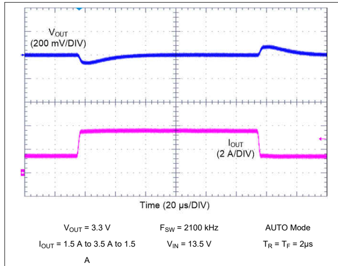
图 9-23. LM62435-Q1 Load Transient
