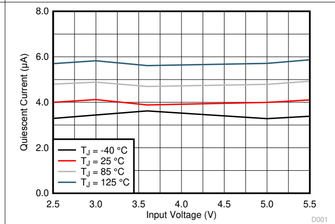
图 7-4. Quiescent Current
