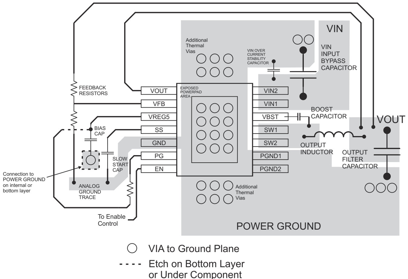
图 15-1. PCB Layout
