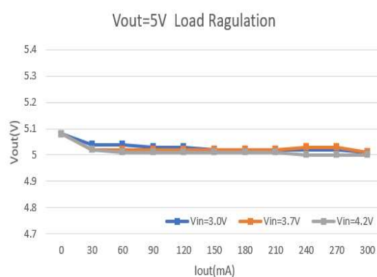
图 4. Load Regulation
