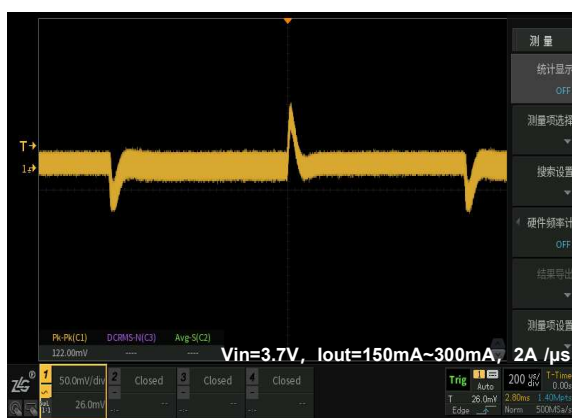
图 5. Load Transient
