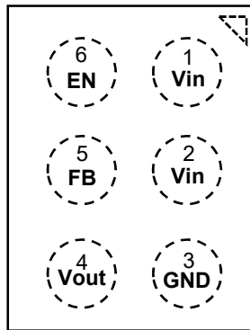
图2.顶视图 (透视)
