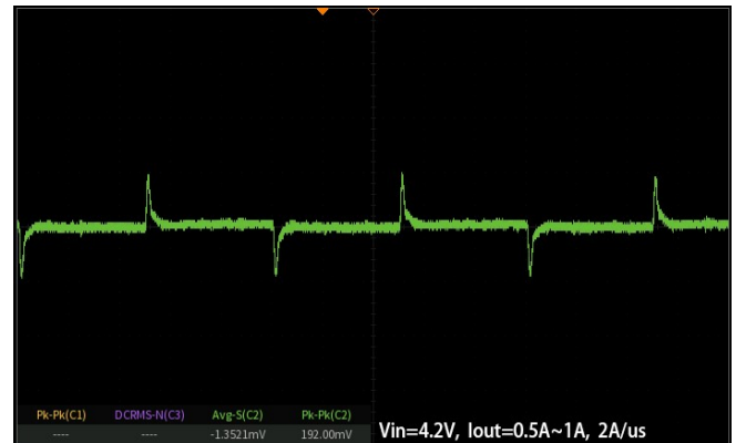
Vin=4.2V 动态响应
