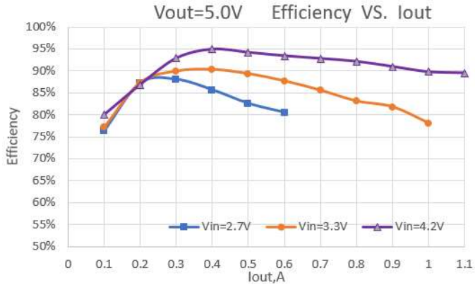
效率
