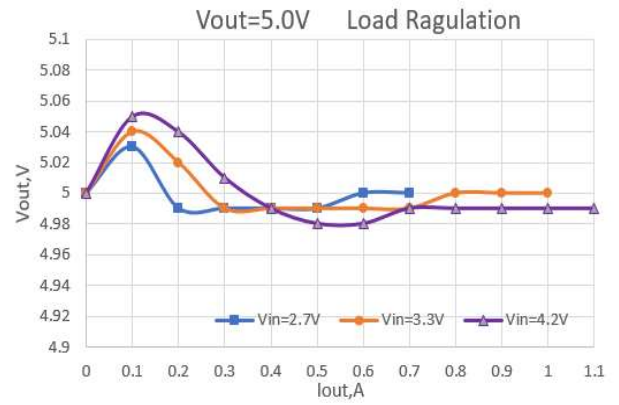
负载调整率
