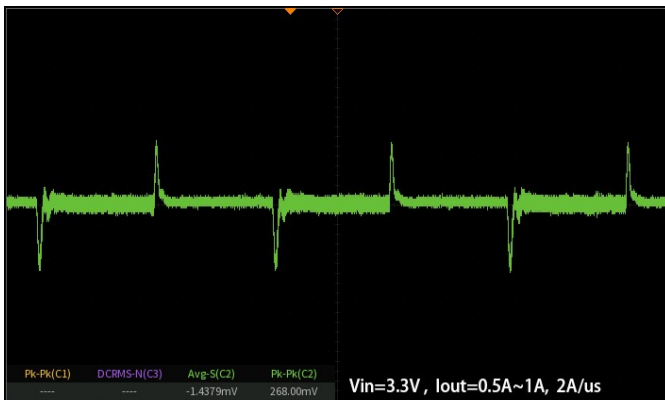
Vin=3.3V 动态响应
