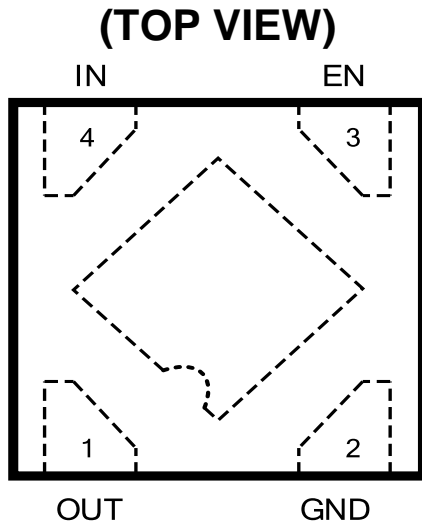
UTDFN-1x1-4
