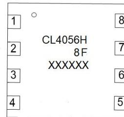
DFN3*3-8L
