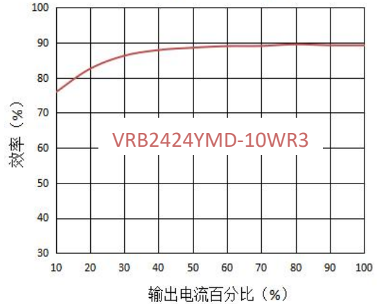
输出效率vs输出负载（24V输入）
